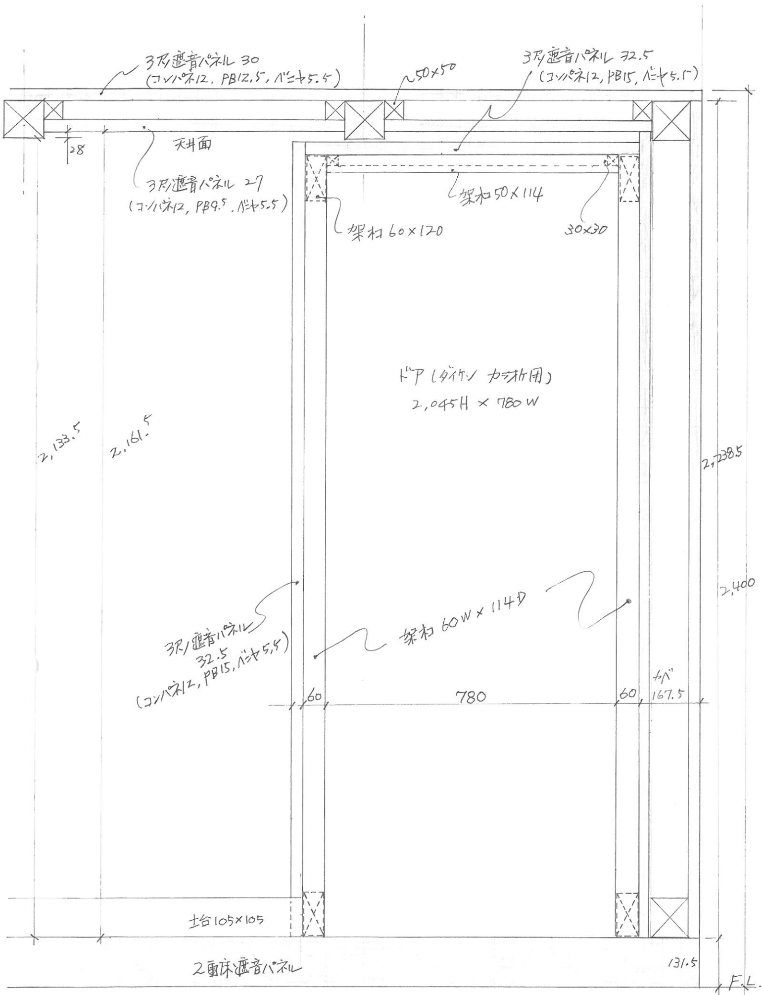
バンド練習室入口断面図 SCALE: 1/10
